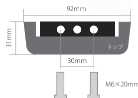
取付ステー
