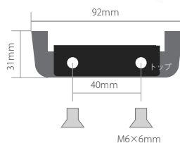
取付ステー
